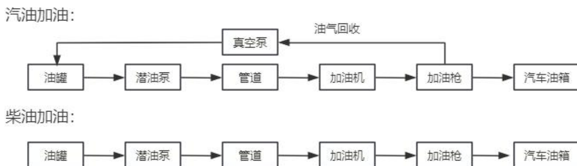
图 2.5-2 加油工艺流程图
