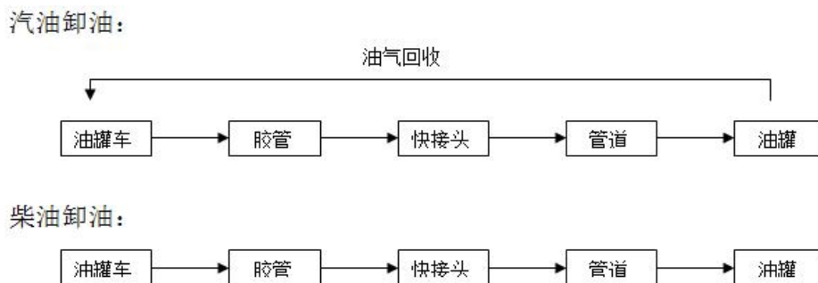
图 2.5-1 卸油工艺过程图
